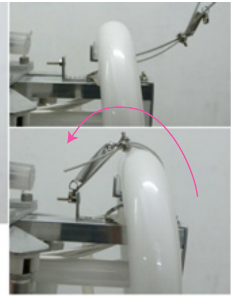
4.9wランプを専用の取り付け器具上に乗せ、器具付属のワイヤ先端のリングをネジに引っ掛けます。
