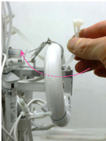
5.6.7.ワイヤでランプを固定した後、さらにランプを安定させるため結束バンドを使用します。器具の2本の脚（ネジ）の奥部分のリングに結束バンドを通し、結束バンドでランプを固定します。 *結束バンドはリユース可能タイプで、爪を押すとバンドを外すことができます。
