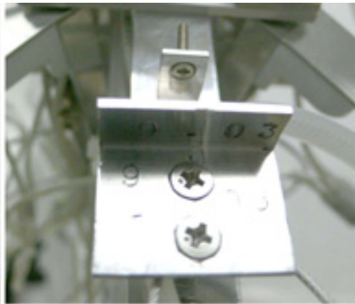
2/3.9wランプ固定用金具に「9-03」「9-06」と2つの刻印があるのは、この位置では9wランプを上下に2段連結してセットするという意味。 *「9-02」のように、刻印が1つの表示の個所ではランプが1つになります。
