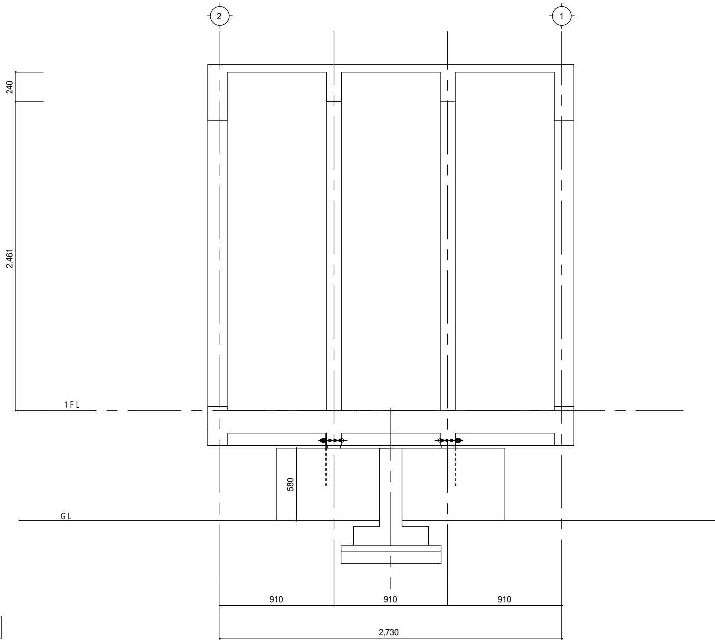
断面图
