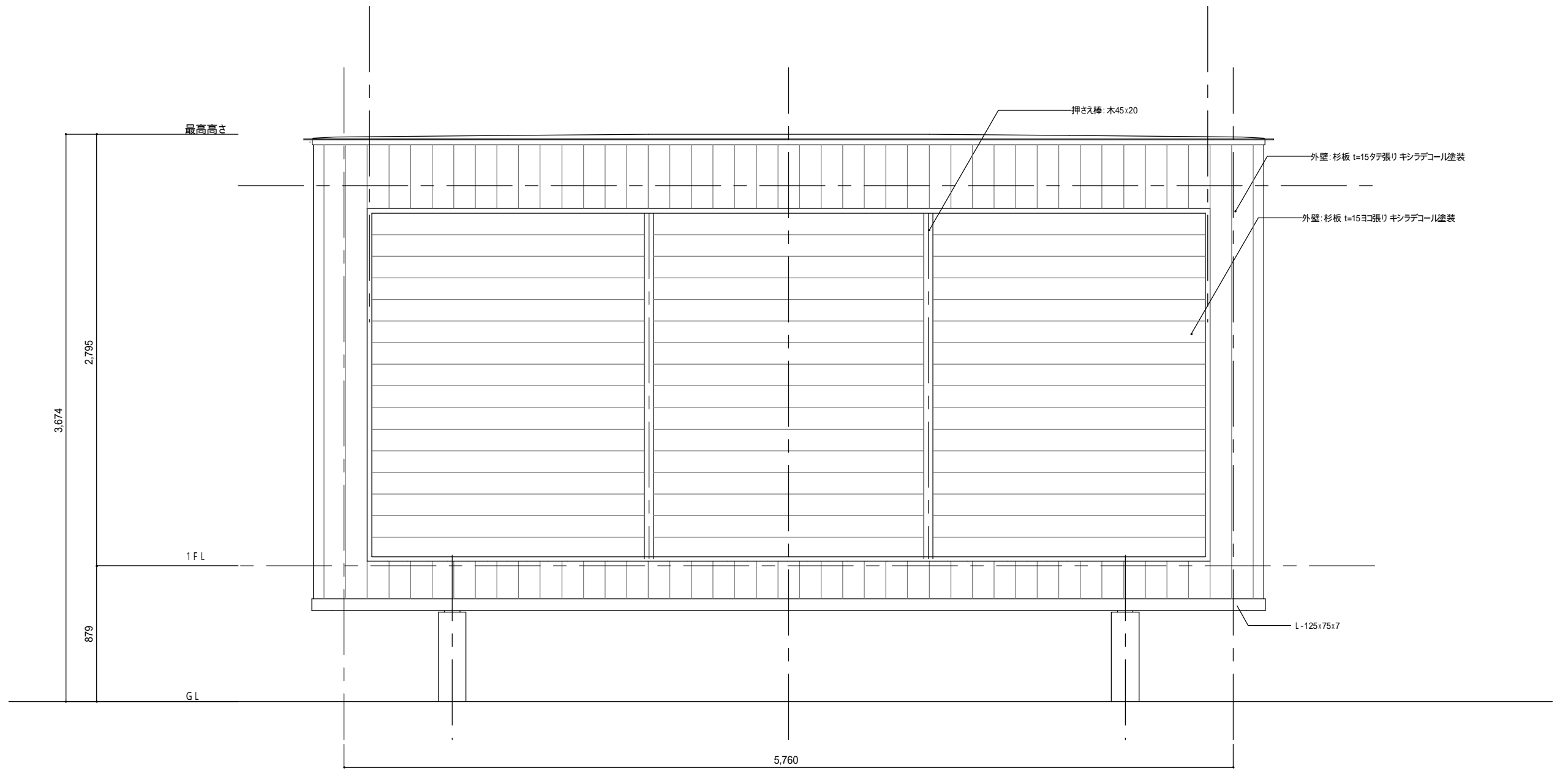
立面図
