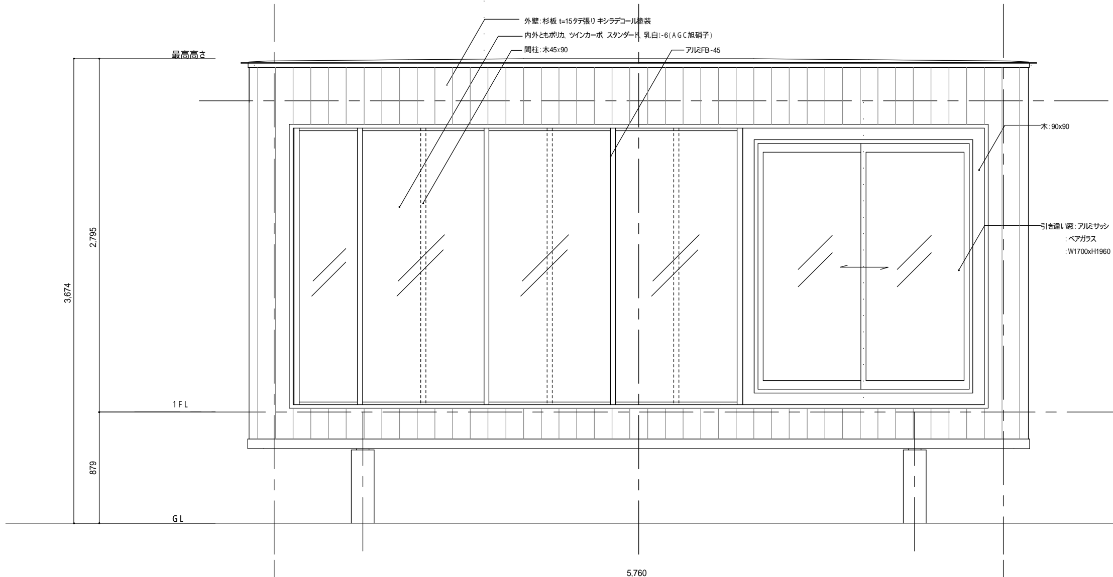
立面図
